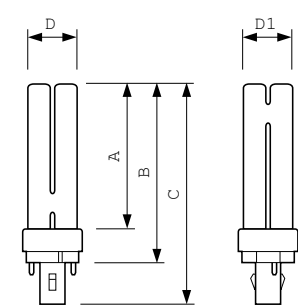
PL-C 10W/827/2P
