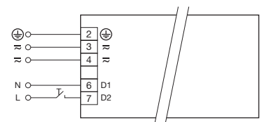
switchDIM PCA T5 EXCEL one4all Ip xitec II
