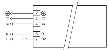
corridorFUNCTION PCA T5 EXCEL one4all Ip xitec II
