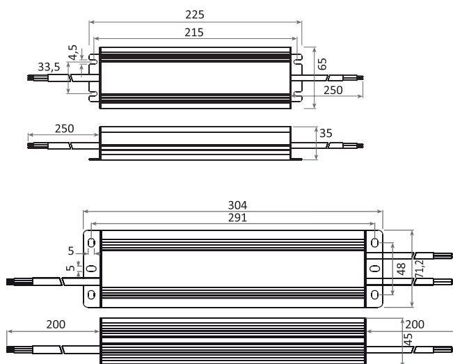
Schémas techniques
