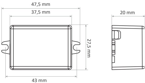
Schéma technique
