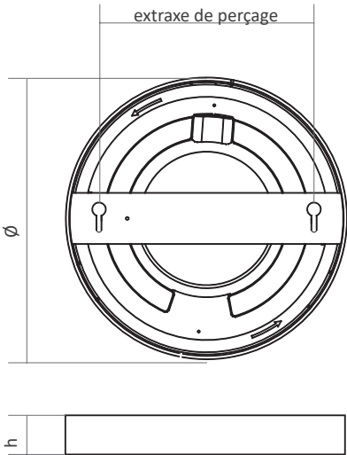
Schéma technique
