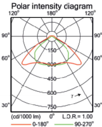
DISTRIBUTION DE LA LUMIÈRE DIFFUSEUR TRANSPARENT
