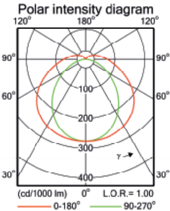
DISTRIBUTION DE LA LUMIÈRE DIFFUSEUR OPALE
