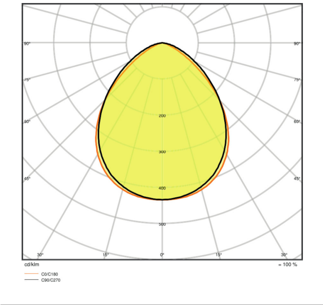
Courbe photometrique, polaire
