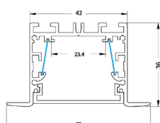
Profil pour SKYLINE encastré
