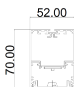
Profil pour SKYLINE saillie et suspendue
