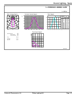
LEDspots MAS SLR 14,8W AR111 G53 940 45D-ADL ADL
