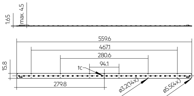
LLE 16x560mm 2400lm HV ADV6
