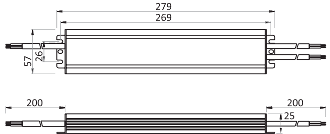
Schéma technique
